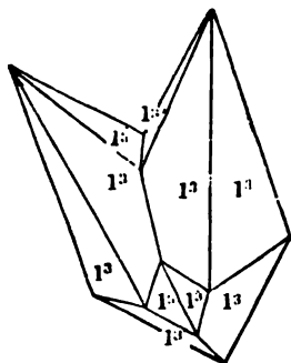
Calcite.
